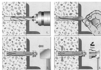
Abb. 4: Einbauanleitung Segmentanker
