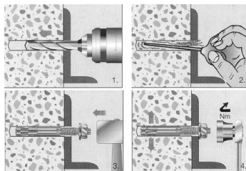
Abb. 4: Einbauanleitung Segmentanker
